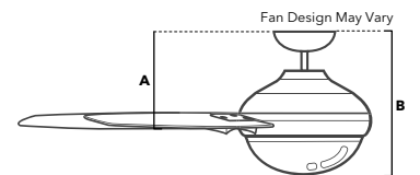
Fan Dimensions in Centimeters
