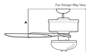
Fan Dimensions in Centimeters
